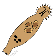
Dactylogyrus.
